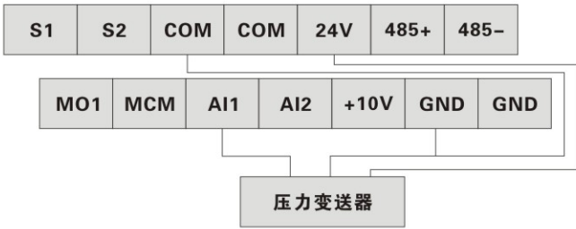
三线制压力变送器接线图
