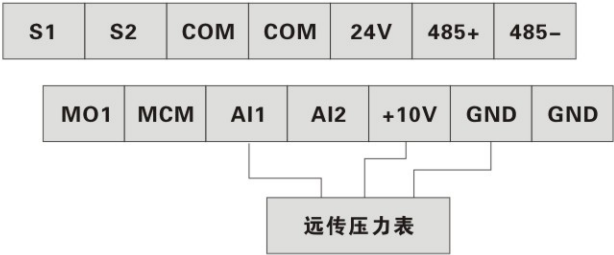
远传压力表接线图
