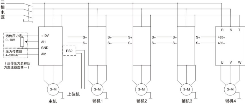
端子接线图 (最多可控制5台辅机)
