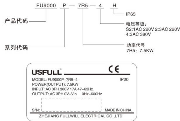
图 1-2 变频器铭牌说明
