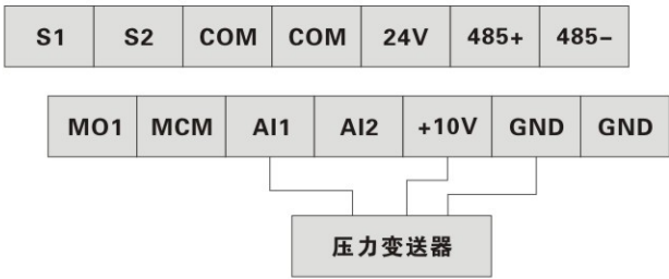
三线制压力变送器接线图
