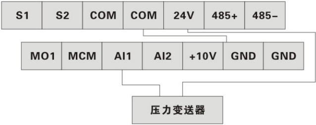
远传压力表接线图
